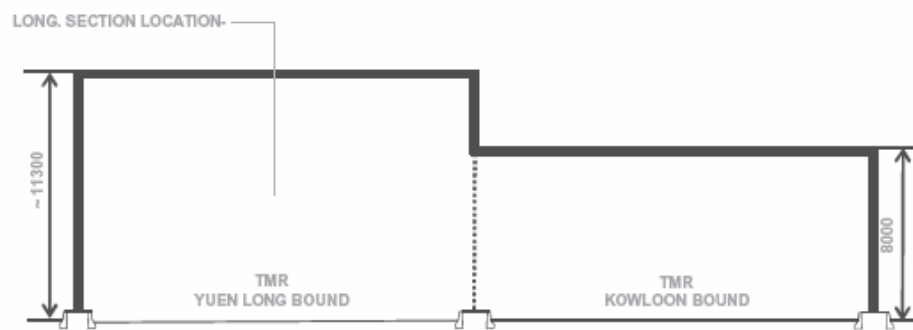
SECTION 12-12 FULL ENCLOSURE NM 19 (N.T.S.)
