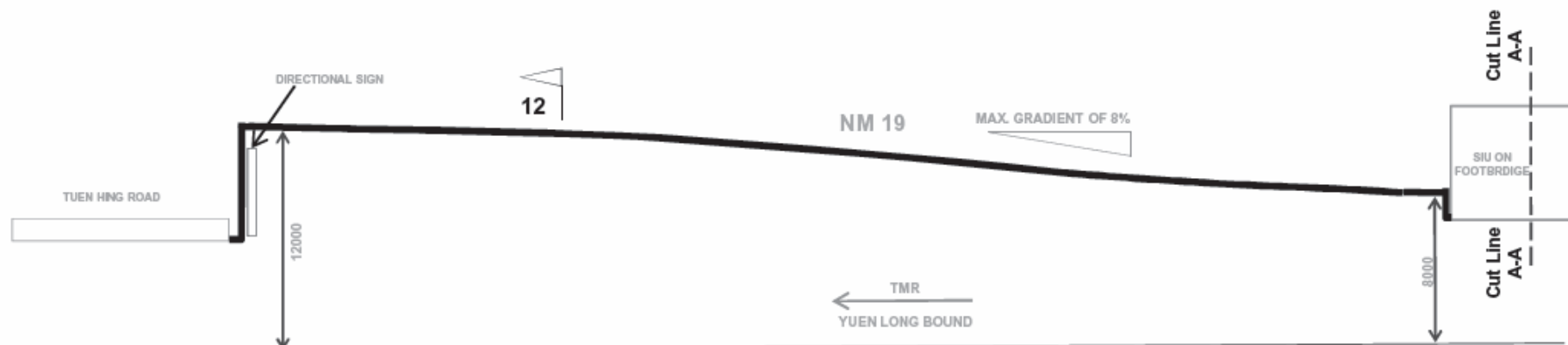
12 LONGITUDINAL SECTION ALONG TMR YUEN LONG BOUND AT NM19 (N.T.S.)
